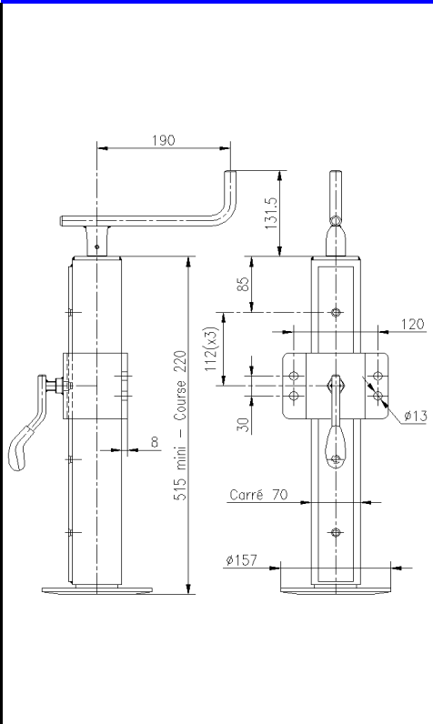
1200825 BÉQUILLE Carré 70 Charge statique = 350kg (Poids : 12,6kg)
