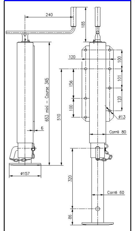
1200835 BÉQUILLE Carré 80(*) Charge statique = 1000kg (Poids : 21,4kg)
