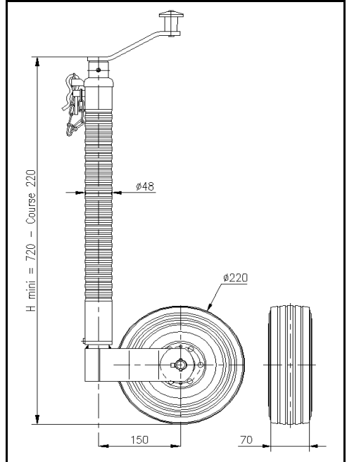
1200358 COULISSEAU Ø48 Pour roue jockey à gorges
