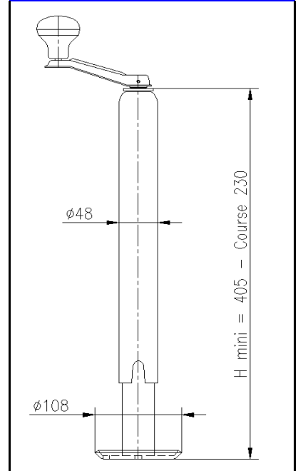
En OPTION: 1200222 COULISSEAU Ø48
