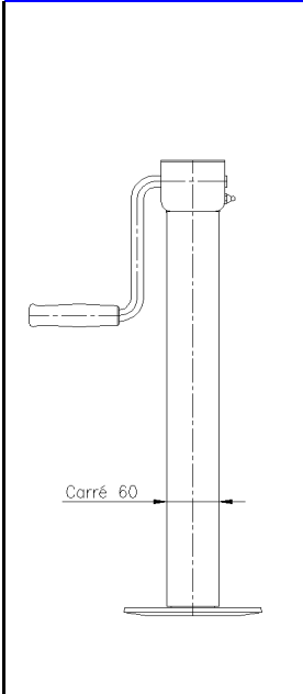
1200393 (voir 1200394) SANS SUPPORT
