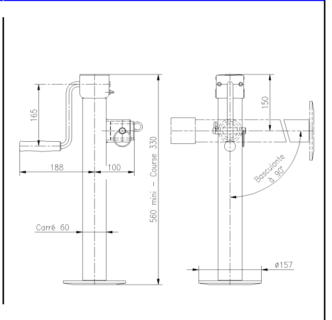
1200394 BÉQUILLE Carré 60 Charge statique = 200kg AVEC SUPPORT ==> BASCULANTE (Poids : 9,2kg)
