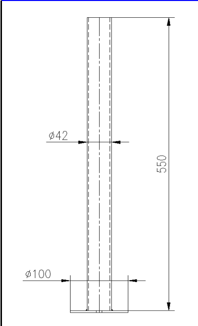
En OPTION: 1200027 COULISSEAU Ø42
