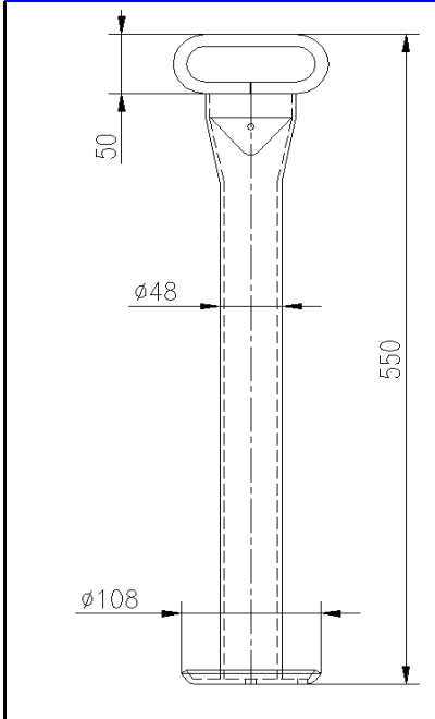
En OPTION: 1200222 COULISSEAU Ø48
